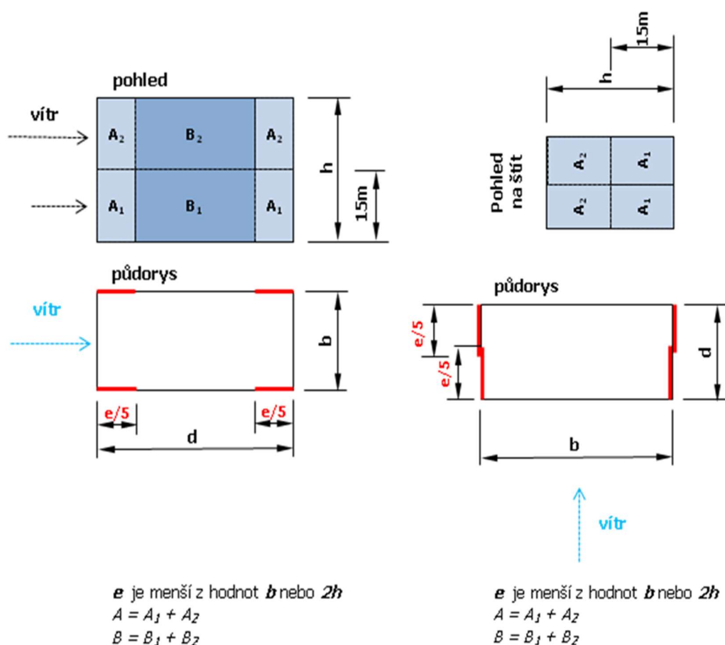
Obr. 10: Grafické znázornění jednotlivých parametrů pro stanovení okrajové a vnitřní oblasti plochy
