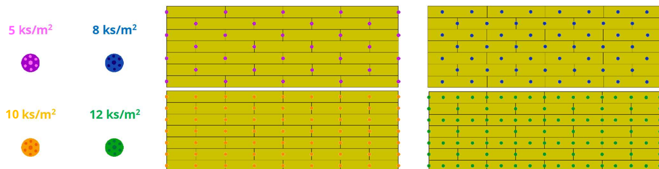
Obr. 9: Příklad rozmištění kotvicích hmoždinek desky-lamely 200×1 000 mm (200×1 200 mm)
